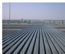
Juntas modulares
